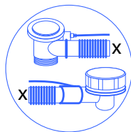
Överflylnadsskydd m. anslutning till avloppssats Beställningsnr. 8000-110-3501
