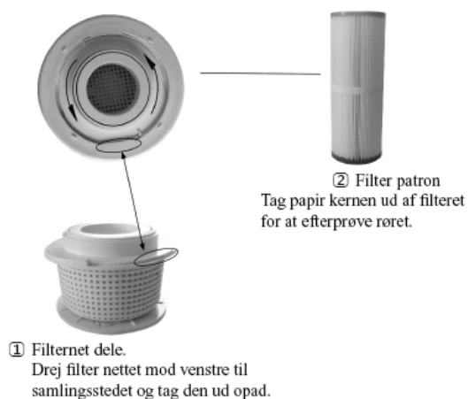
Tegning 1: Fremgangsmåden at skifte filter patronen
